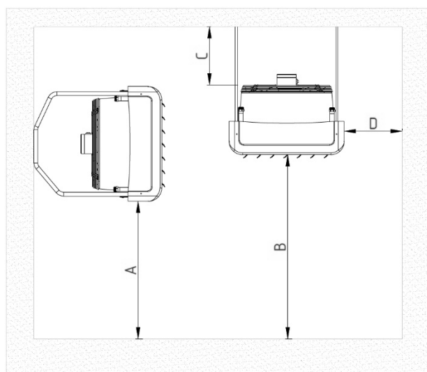
Рис. 1. Рекомендуемые расстояния для монтажа
