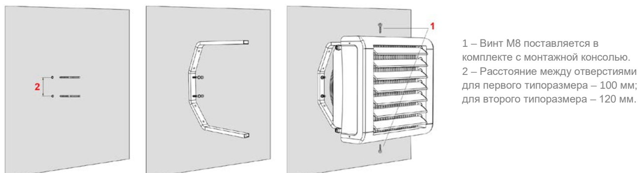
Рис. 4. Монтаж консоли
