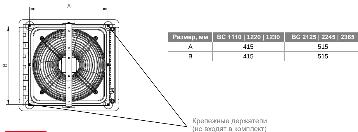
Рис. 2. Расстояния между крепежными держателями
