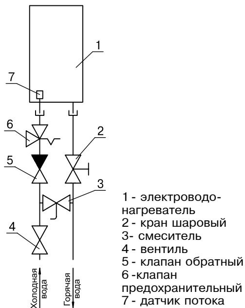
Рис.5 Схема гидравлическая принципиальная
